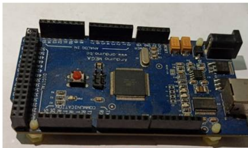
Arduino Mega
